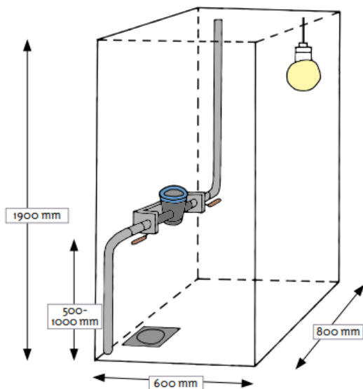
Mätarplatsens utformning med minsta godkända mått för att mätarplatsen ska kunna godkännas.
